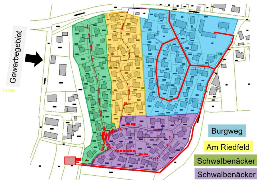
Nahwärmeleitung - Konzept
